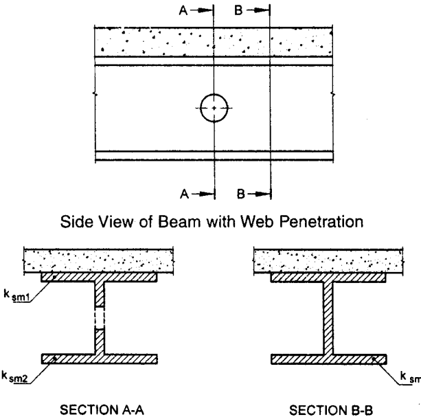
FIG. 26 WEB PENETRATION
